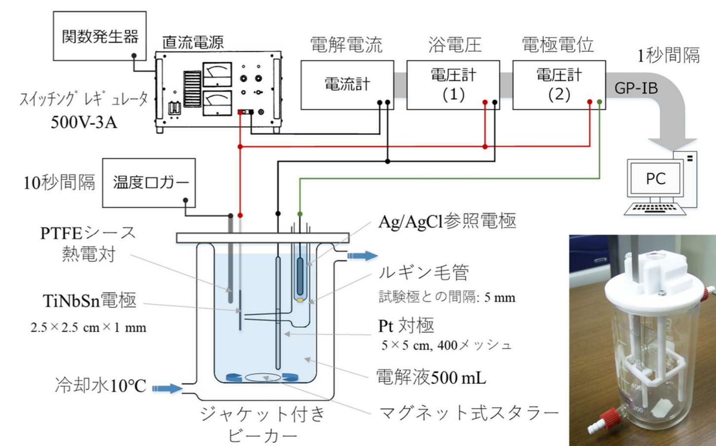
図2 陽極酸化実験に使用するセットアップ → 高圧印加可能な水冷ジャケット電気化学セル
