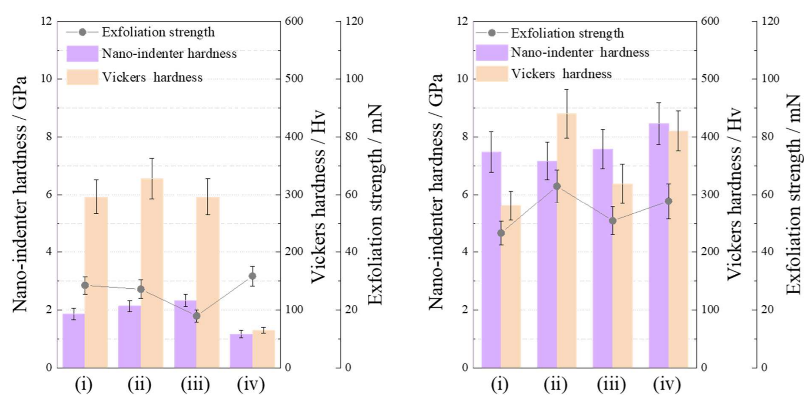
図3 陽極酸化Ti6Al4V (左) とTiNbSn (右) 合金の硬度と基板密着強度 → 硬度も密着強度もTiNbSn基板陽極酸化材がTi6Al4V基板材より高い
