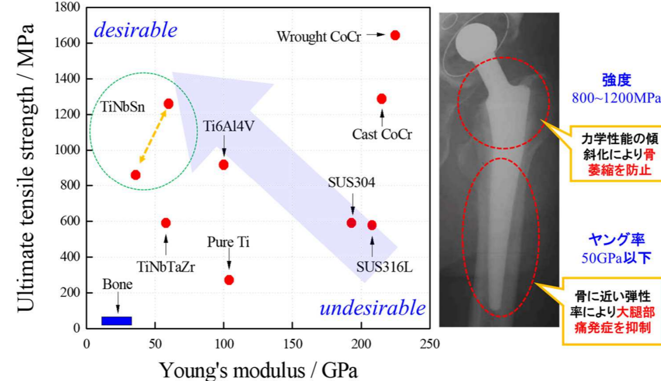
図1 金属系バイオマテリアルの引張強度とヤング率の相関 → TiNbSn合金は同一素材で高強度部と低ヤング率部を兼備
