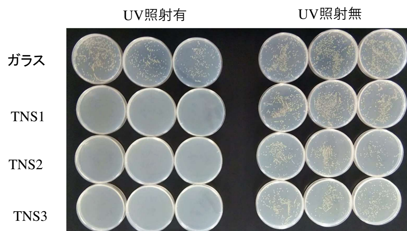
図7 陽極酸化TiNbSn合金とガラス (コントロール) に対して行った寒天培地に生えた菌コロニー
