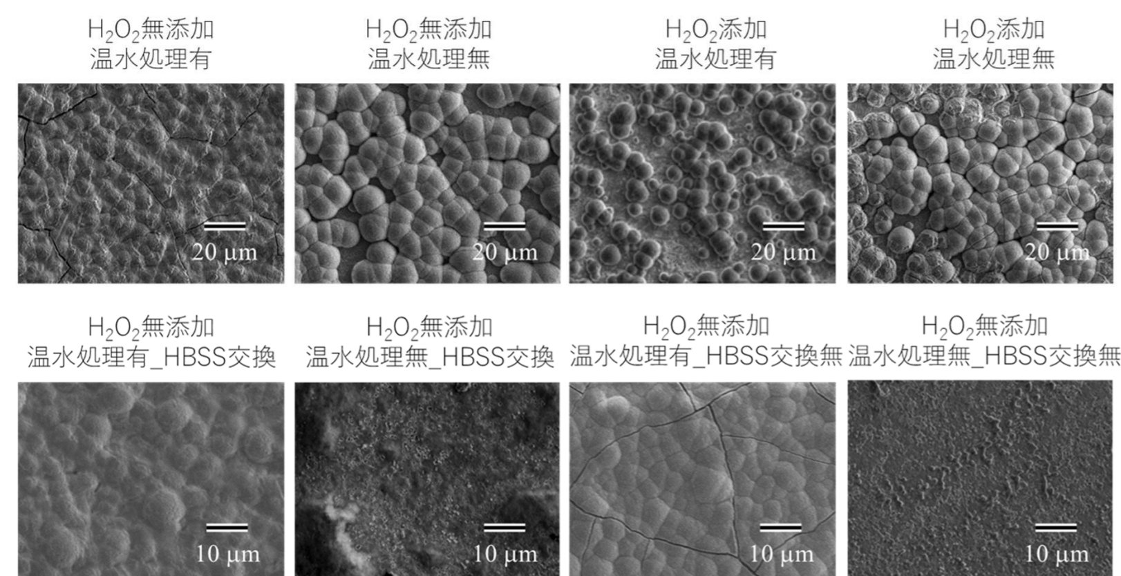
図6 各種処理を施した陽極酸化TiNbSn合金を疑似体液浸漬後のハイドロキシアパタイト析出を示すSEM像
