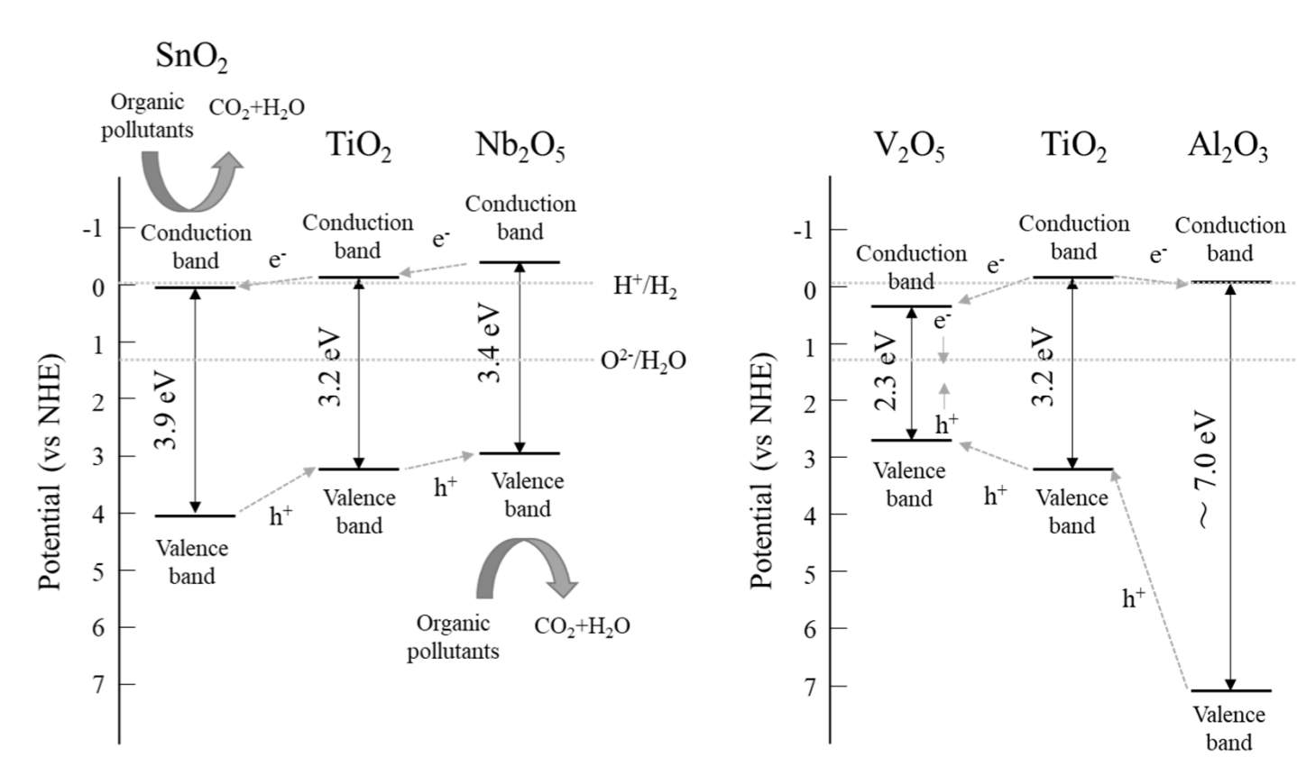
図11 陽極酸化TiNbSn (左) とTi6Al4V (右) のヘテロジャンクションモデル模式図
