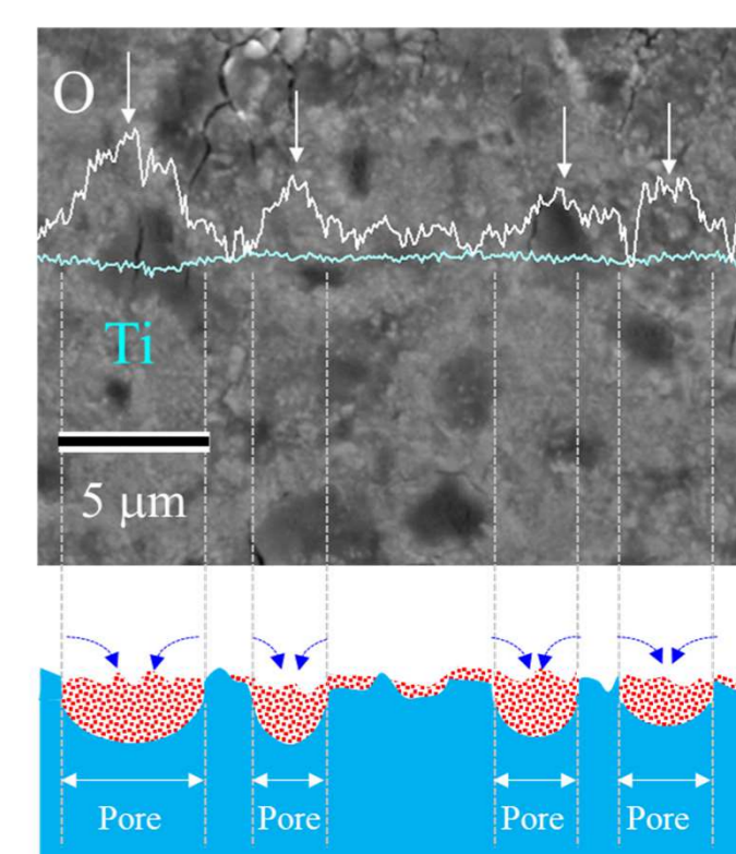
図5 TiNbSnの湿潤摩耗試験後のSEM像 (上) と物質移動図 (下)
