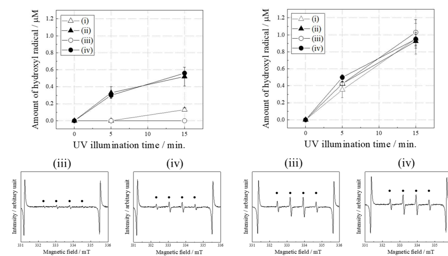
図10 陽極酸化Ti6Al4V (左) とTiNbSn (右) のヒドロキシラジカル生成量の照射時間依存性とESRスペクトル
