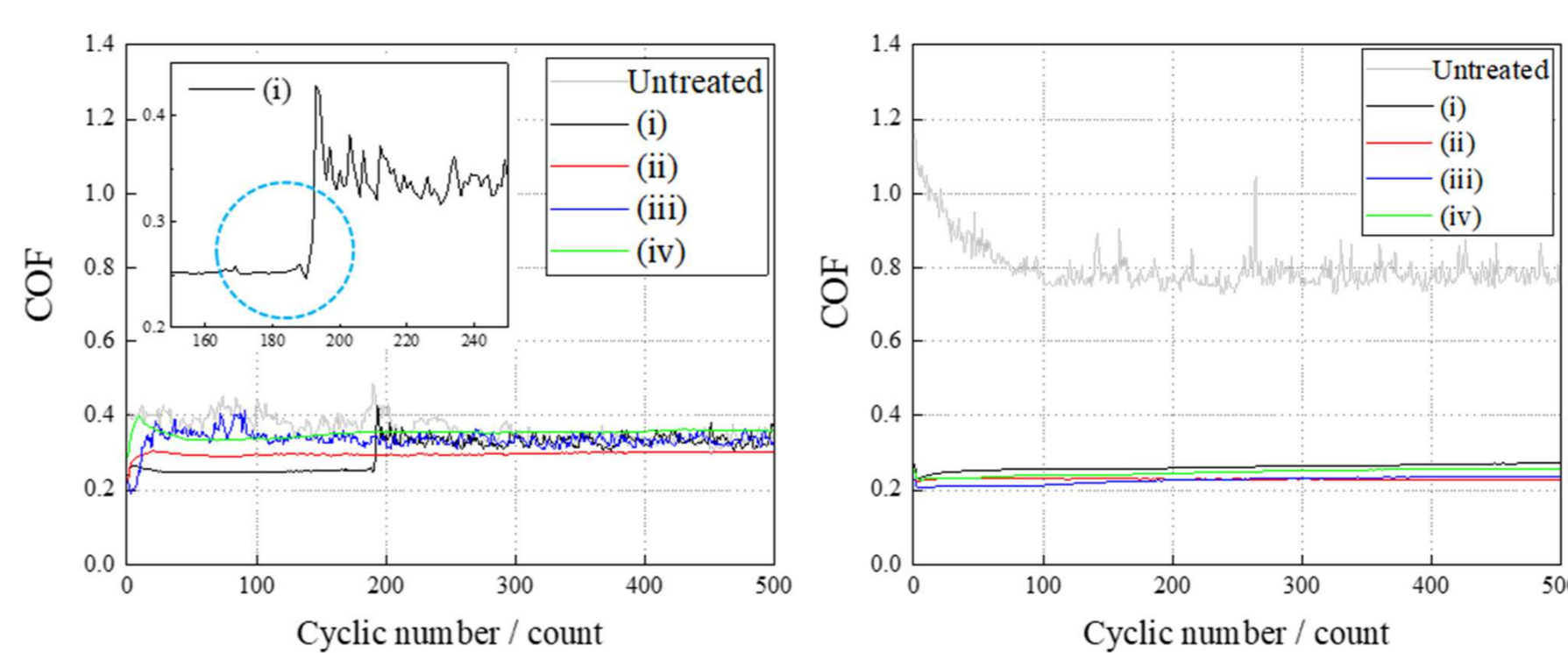
図4 陽極酸化Ti6Al4V (左) とTiNbSn (右) の湿潤下での摩耗試験 → 摩擦係数はTiNbSn基板陽極酸化材の方が低く安定に推移する
