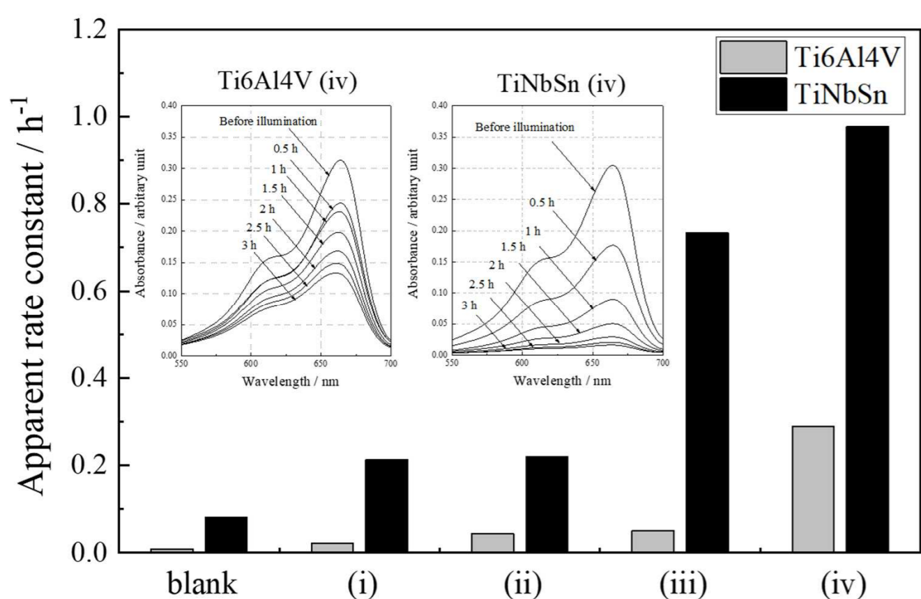
図9 陽極酸化TiNbSnとTi6Al4VのMB脱色試験に反応速度とMBスペクトルの経時変化
