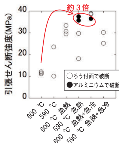
熱処理条件と重ね合わせ継手の引張せん断強度
