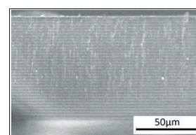
オールカーボン光学多層膜の外観と断面SEM像
