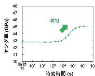
時効処理によるMg-Al合金のヤング率の変化
