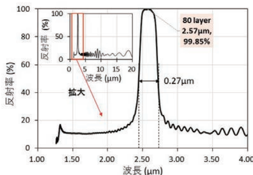
オールカーボン光学多層膜の赤外線波長域の光学反射率
