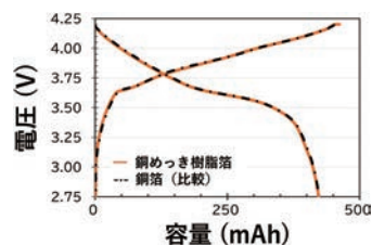
試作電池の充放電特性 (設計容量 440 mAh)
