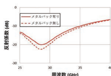
電磁波吸収特性
