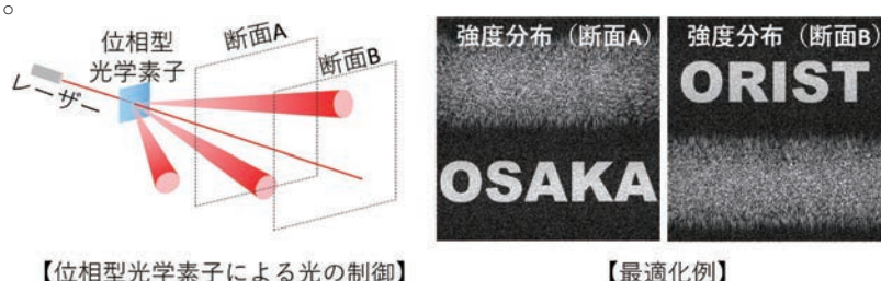
【位相型光学素子による光の制御】
