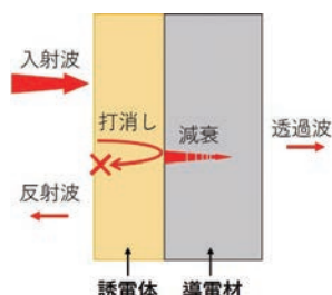
構造模式図
